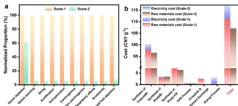
图 3 POPcarbene 吸附剂在不同规模制备下的生命周期评估以及成本分析
